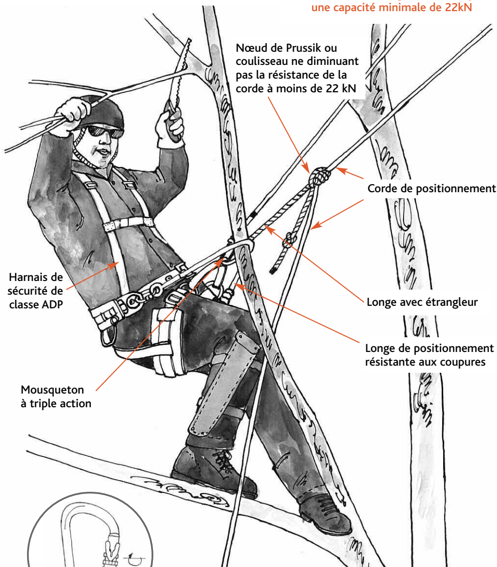
Illustration n° 18 Équipements requis pour les travaux en appui sur corde
