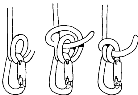
Illustration n° 5 Nœud d'ancre
