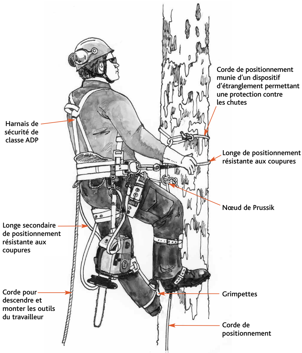
Illustration n° 20 Équipements requis pour le travail à l'aide de grimpettes
