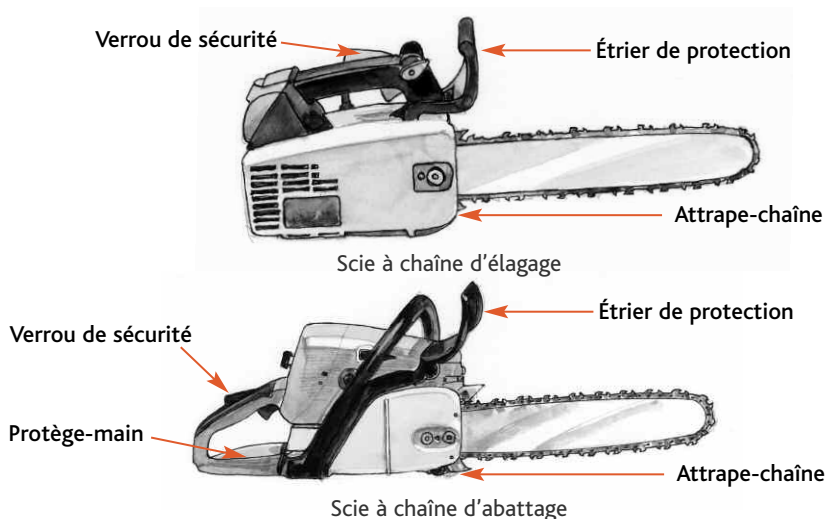
Illustration n° 24 Scies à chaîne d'élague et d'abattage
