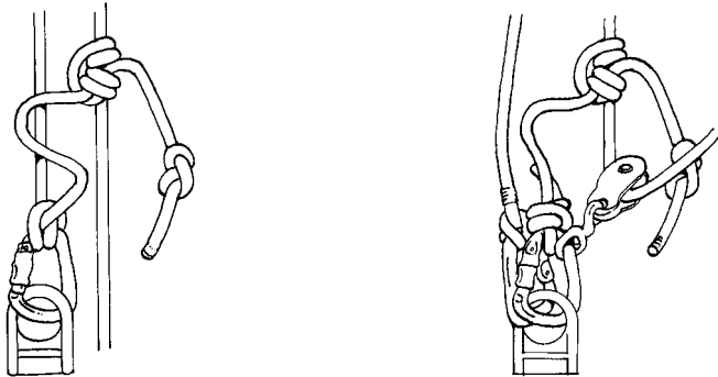
Illustration n° 15 Méthode traditionnelle
