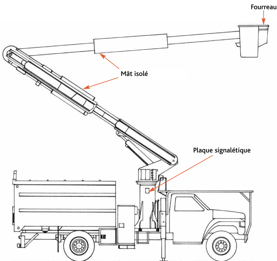
Illustration n° 30 Engin élévateur à nacelle
