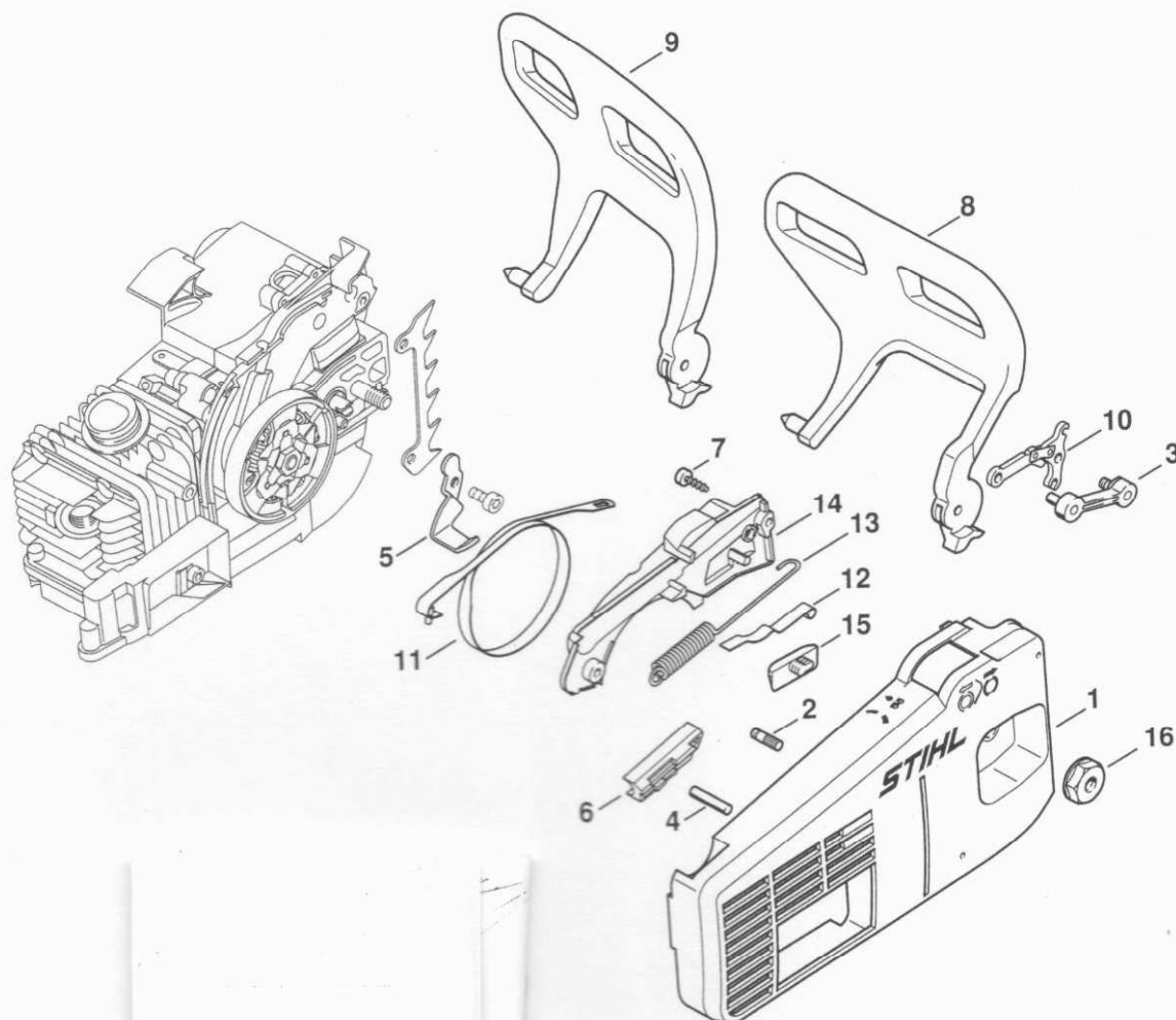
Couvercle de pignon
